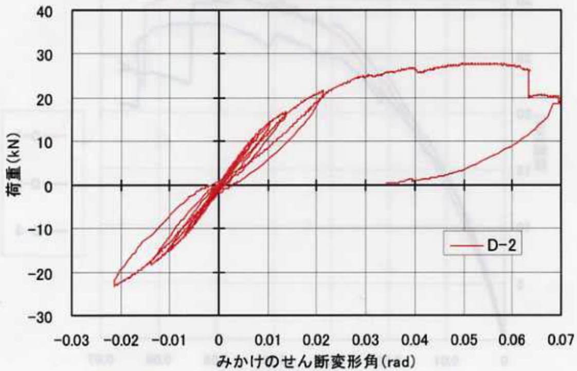
図-3-2 荷重-変形角曲線(D-2)
