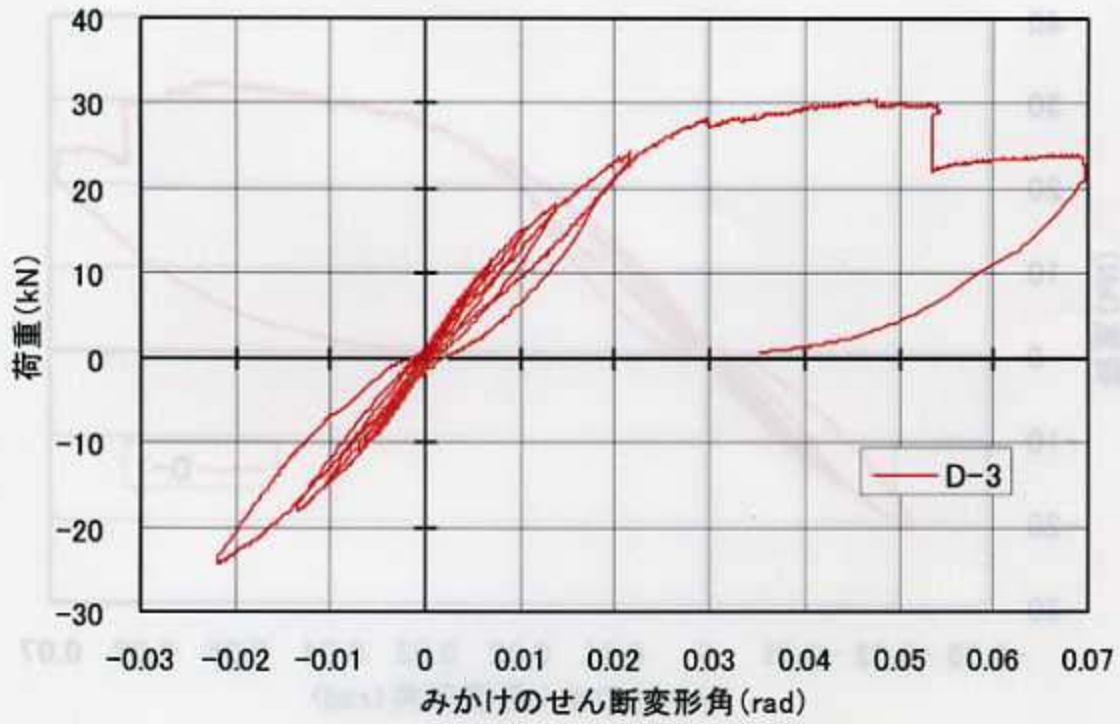
図-3-3 荷重-変形角曲線(D-3)
