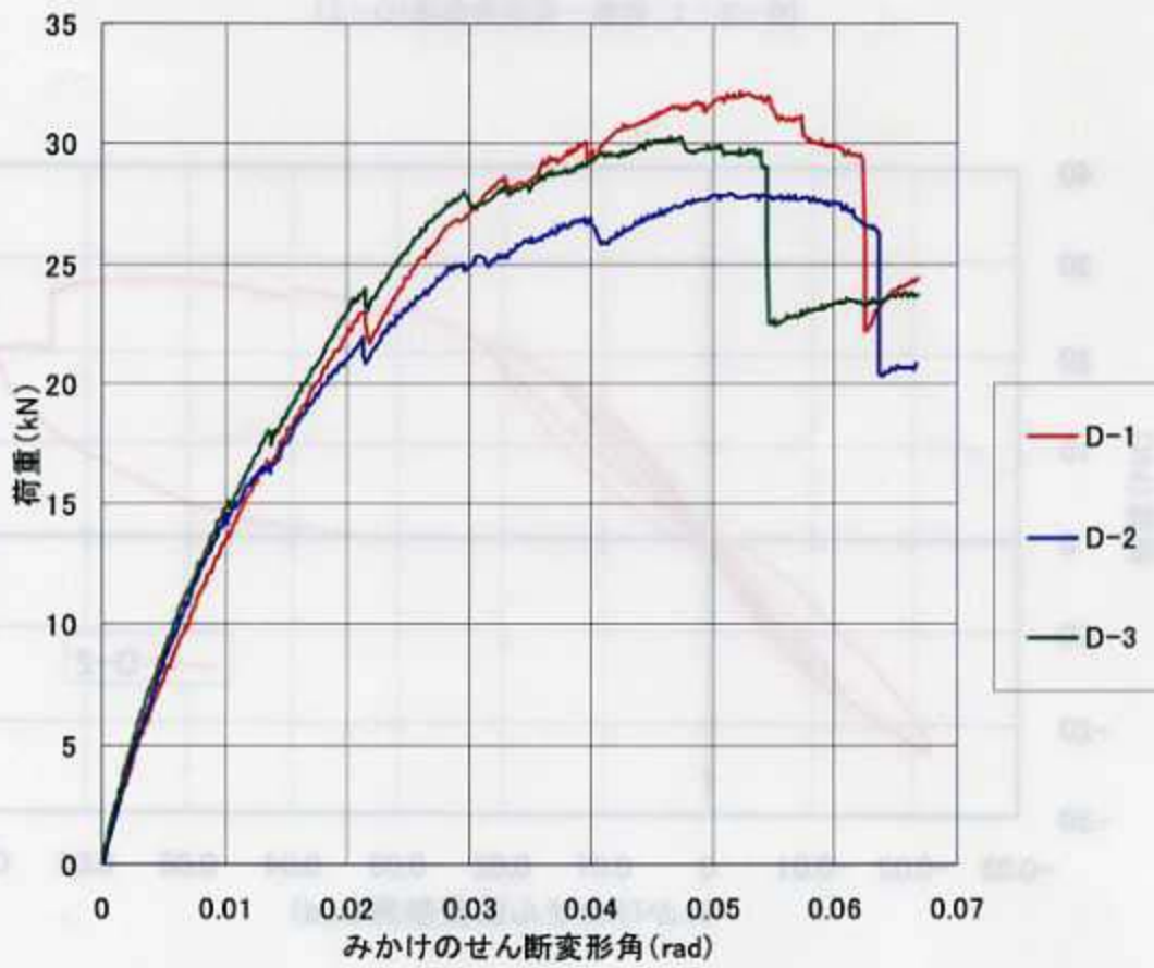
図-4 荷重-変形角包絡線
