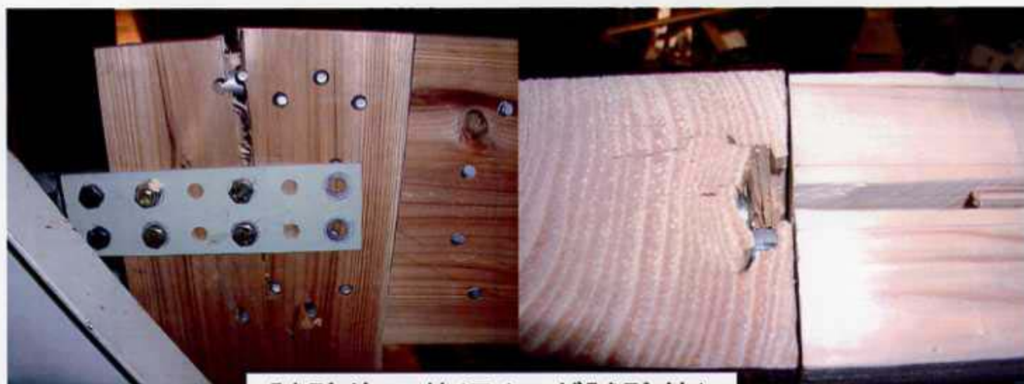
試験後の状況(スギ試験体)
